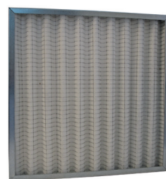
Filtri aria con setto acrilico o metallico. Costruiti in lamiera zincata o in acciaio inox
